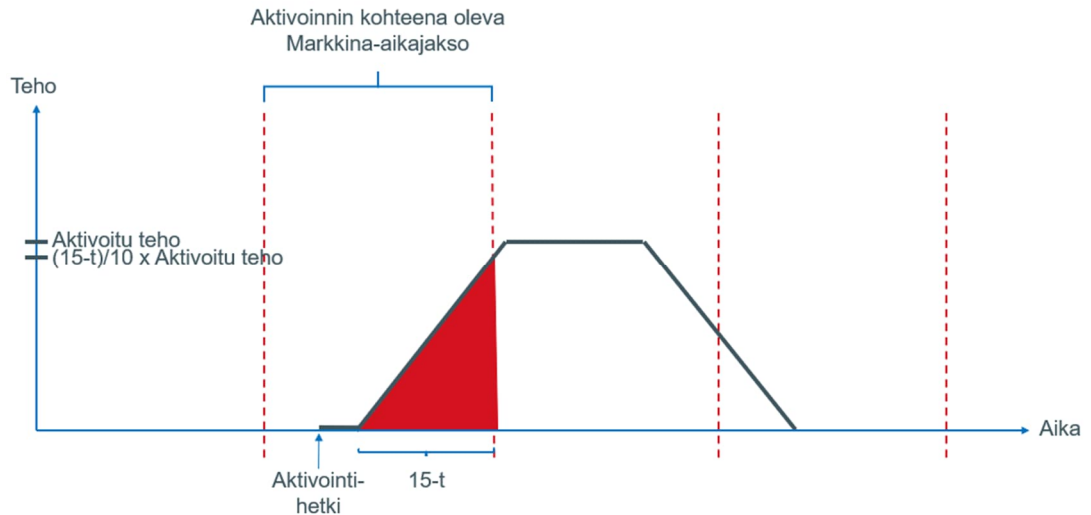
Kuva 10 Suoran aktivoinnin kohteena olevaa Markkina-aikajaksoa vastaavalle Taseselvitysjaksole kohdistuva energia, kun Tehonmuutos alkaa Suoran aktivoinnin kohteena olevan Markkina-aikajakson aikana ja päättyy seuraavalla Markkina-aikajaksolla
