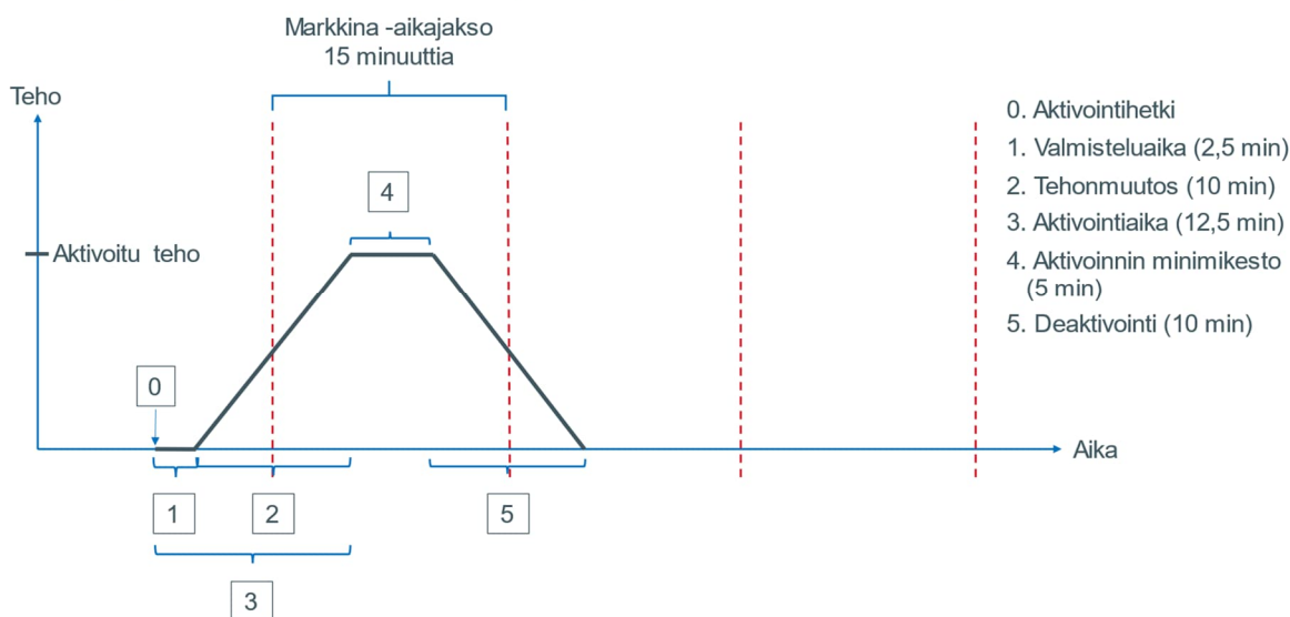
Kuva 1 Ajastetun aktivoinnin periaate 12,5 min aktivointiajalla
