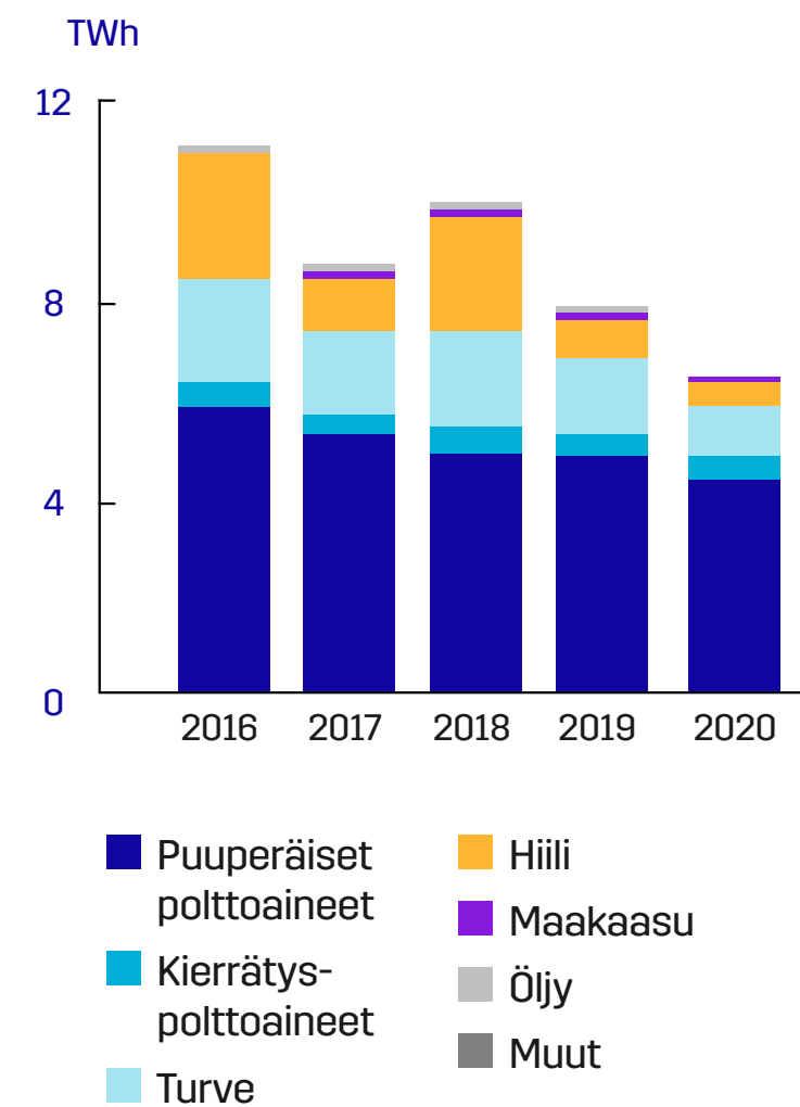
Lämmön- ja sähköntuotannon polttoaineet 2016–2020
